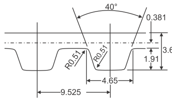
فرم تسمه
