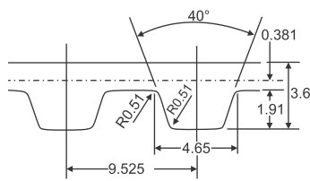
فرم تسمه
