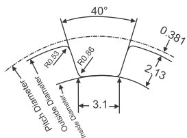
فرم دندانه
