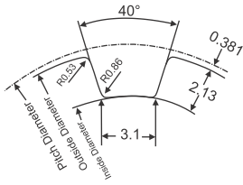
فرم دندان
